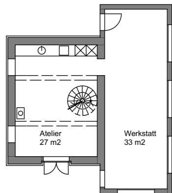
Erdgeschoss 1:200
