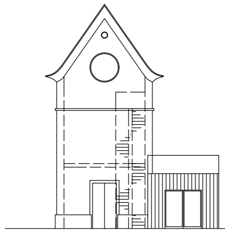
Südfassade 1:200
