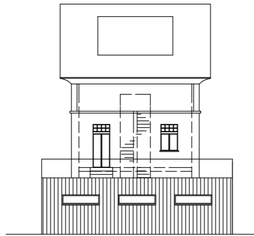
Ostfassade 1:200
