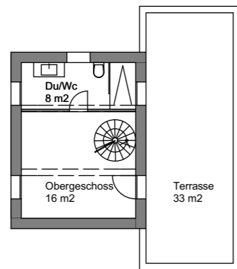
Obergeschoss 1:200
