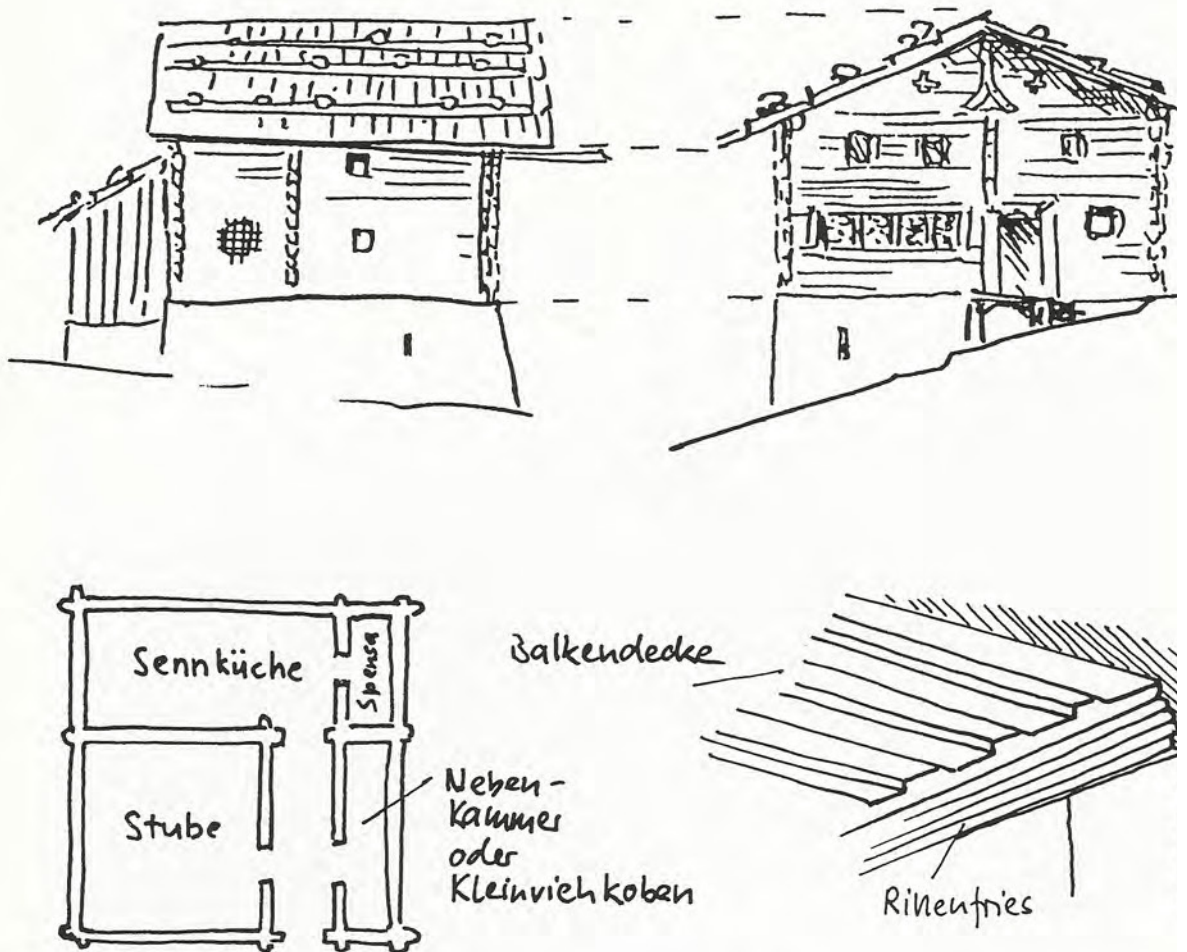
Nesslau, Lutenwil. Ehemaliges Bauernhaus Fiebert. Skizzen des mutmasslichen spätmittelalterlichen Grundbestandes: Ansichten, Grundriss und Stubendecke.
